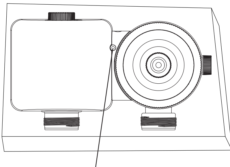
1 x M4 BOULON À TÊTE HEXAGONALE
